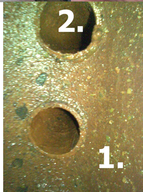
Вскрытые трубы теплообменника после установки витализатора, в конце отопительного сезона. Накипь полностью отсутствует
